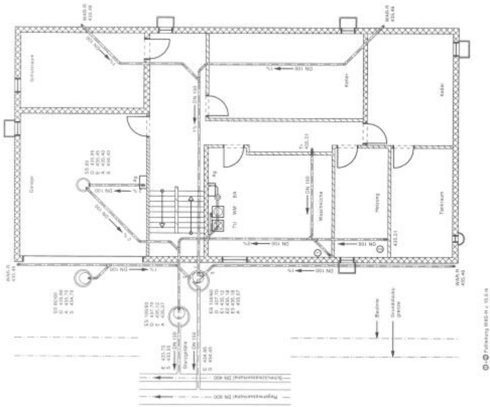
Entwässerungsschema eines Wohnhauses (Trennsystem)
